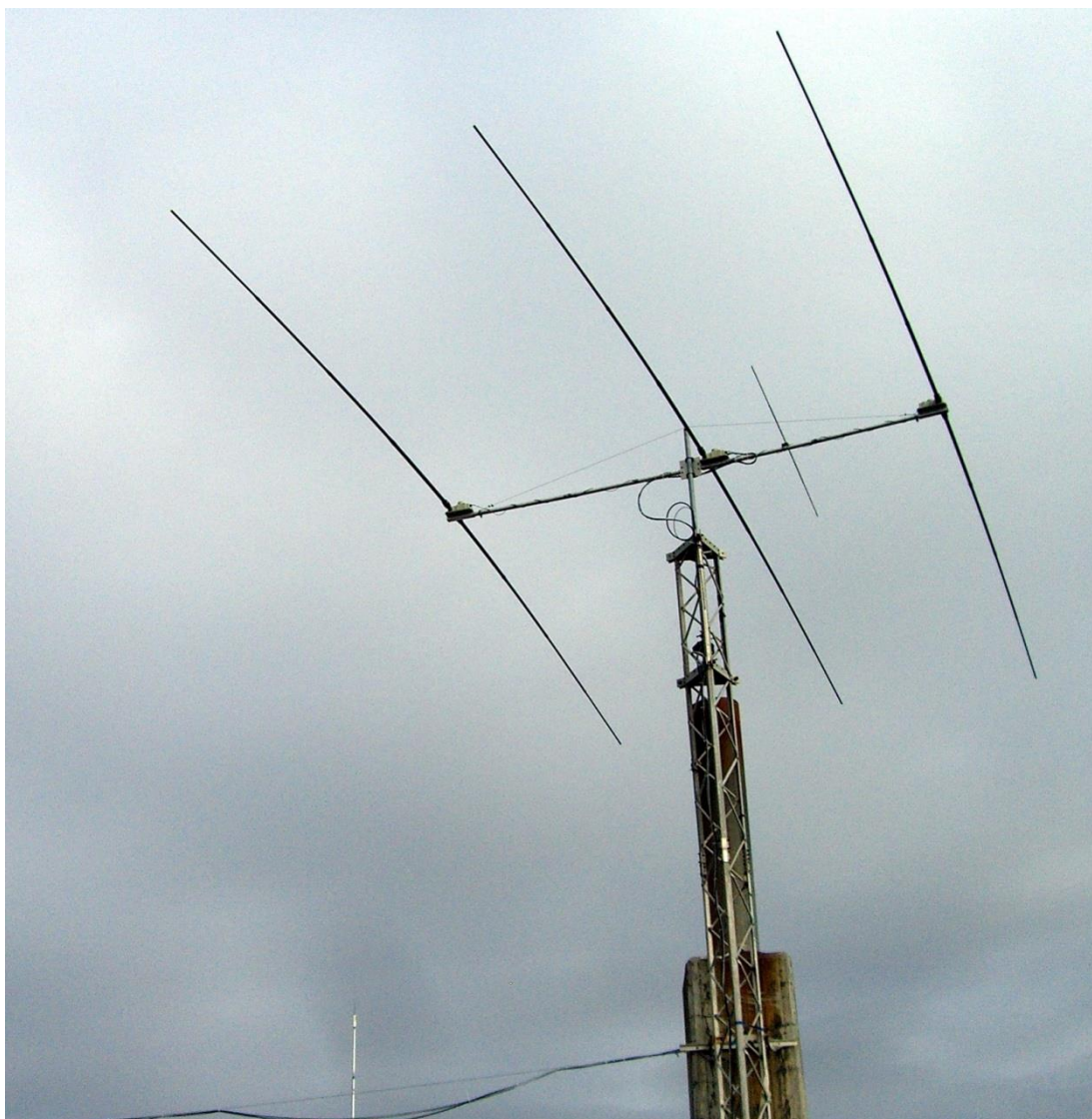
SteppIR 3E Yagi loftnet félagsins vinnur á 6/10/12/15/17/20m. Ef myndin prentast vel má sjá í toppinn á Hustler 6-BTV sem er lóðrétt loftnetsstöng með gildrum (neðst á myndinni til vinstri). Hún vinnur á 10/15/20/30/40/80m. Ljósmynd: TF2JB.
