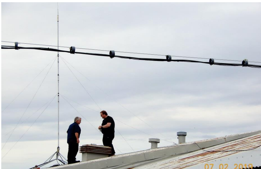
Skeljanesi 2. júlí 2019. Georg Magnússon TF2LL og Guðmundur Sigurðsson TF3GS ganga frá uppsetningu New-tronics Hustler 4-BTV stangarloftnetsins fyrir TF3IRA. Mynd: TF3JB.
